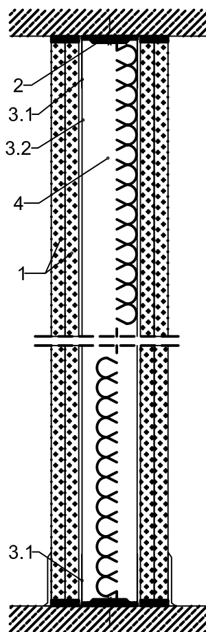
Presek
