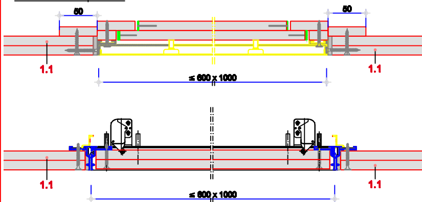
Revizorni otvor Horizontalni presek
