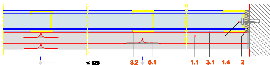
Horizontalni presek
