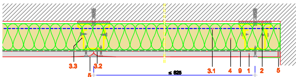
Horizontalni presek
