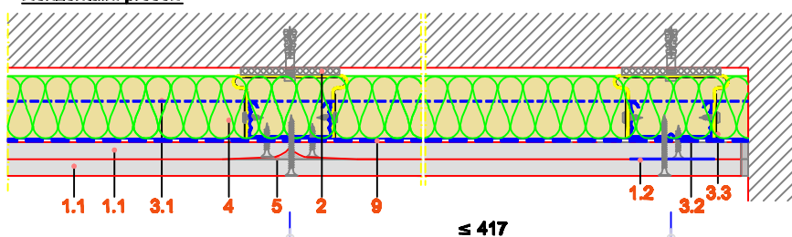
Horizontalni presek
