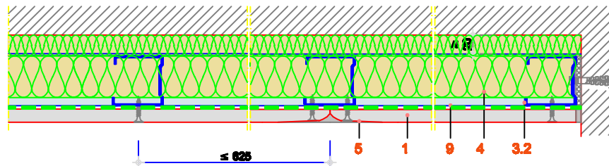
Horizontalni presek
