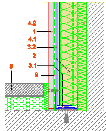
Podni spoj
