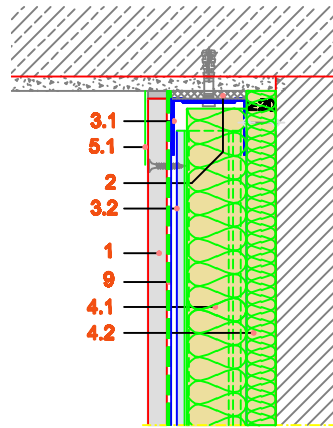
Spoj zida na vlažni malter
