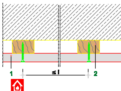
Podužni presek
