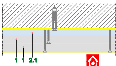
Podužni presek
