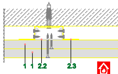
Poprečni presek
