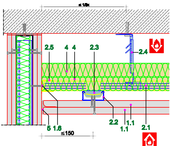
Podužni presek
