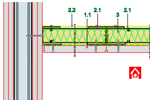
Poprečni presek
