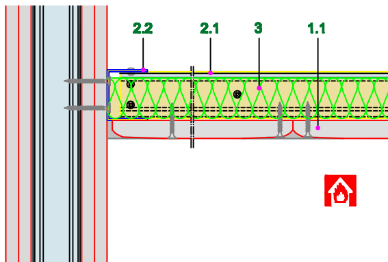
Podužni presek
