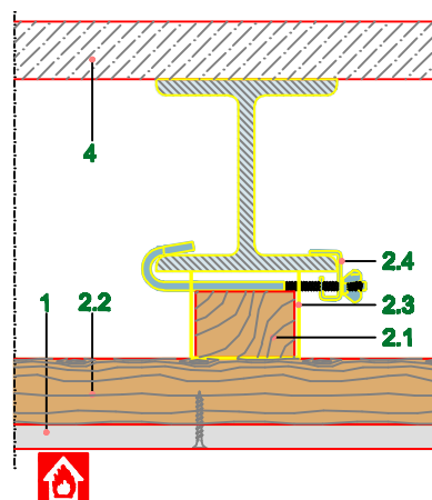
Poprečni presek
