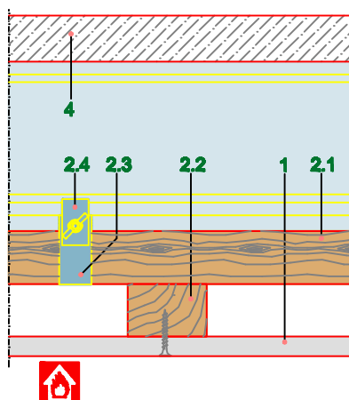
Podužni presek
