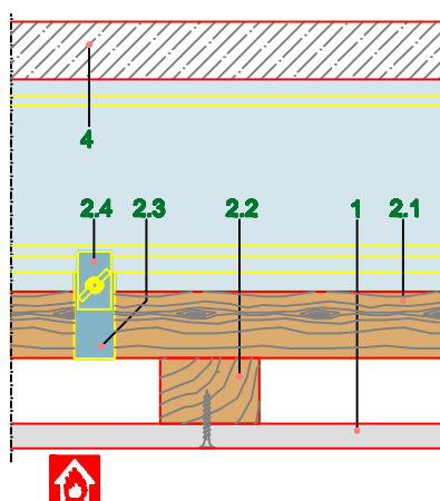
Podužni presek
