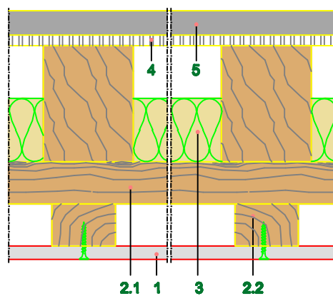
Poprečni presek
