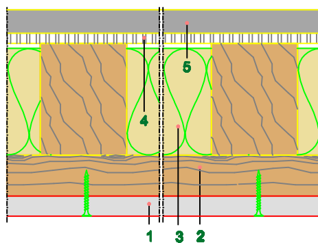
Poprečni presek
