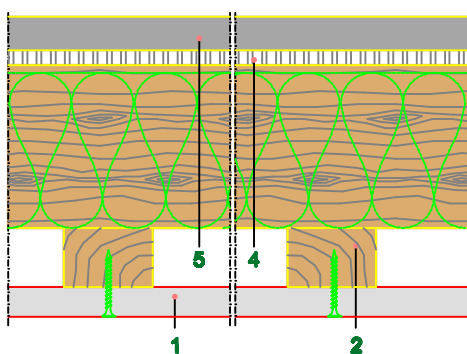
Podužni presek
