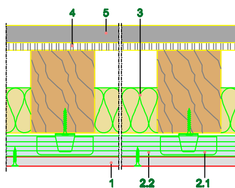
Poprečni presek
