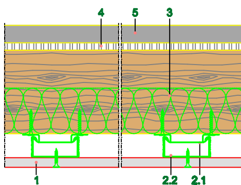
Podužni presek
