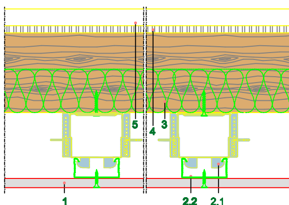
Podužni presek
