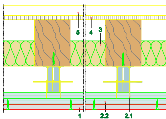
Poprečni presek
