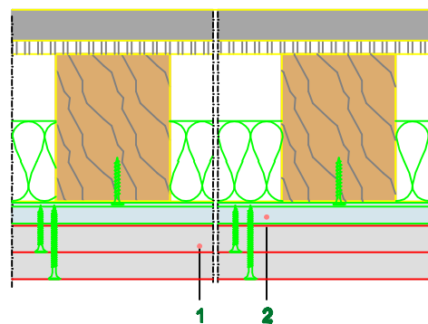
Poprečni presek
