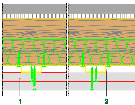
Podužni presek
