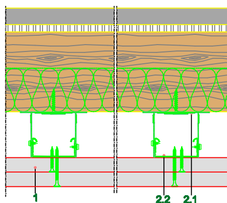
Poprečni presek
