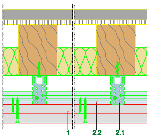
Podužni presek
