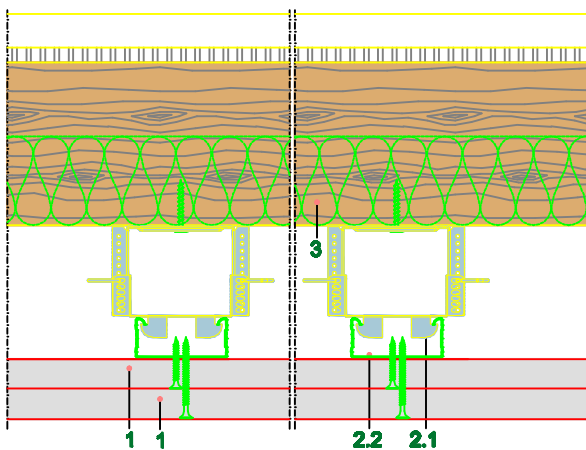
Podužni presek
