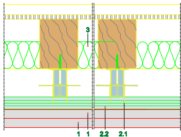
Poprečni presek
