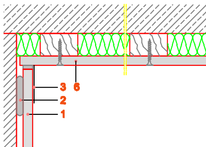
Spoj zida na Rigips plafon
