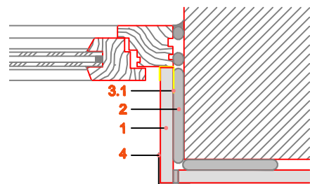
Spoj prozora
