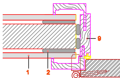
Spoj vrata
