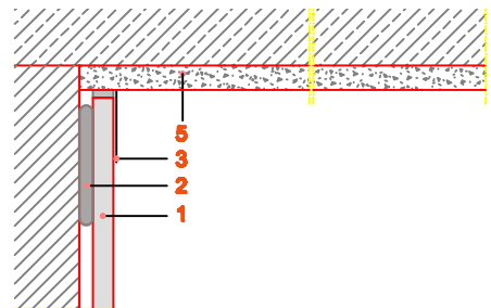
Spoj zida na viažni malter
